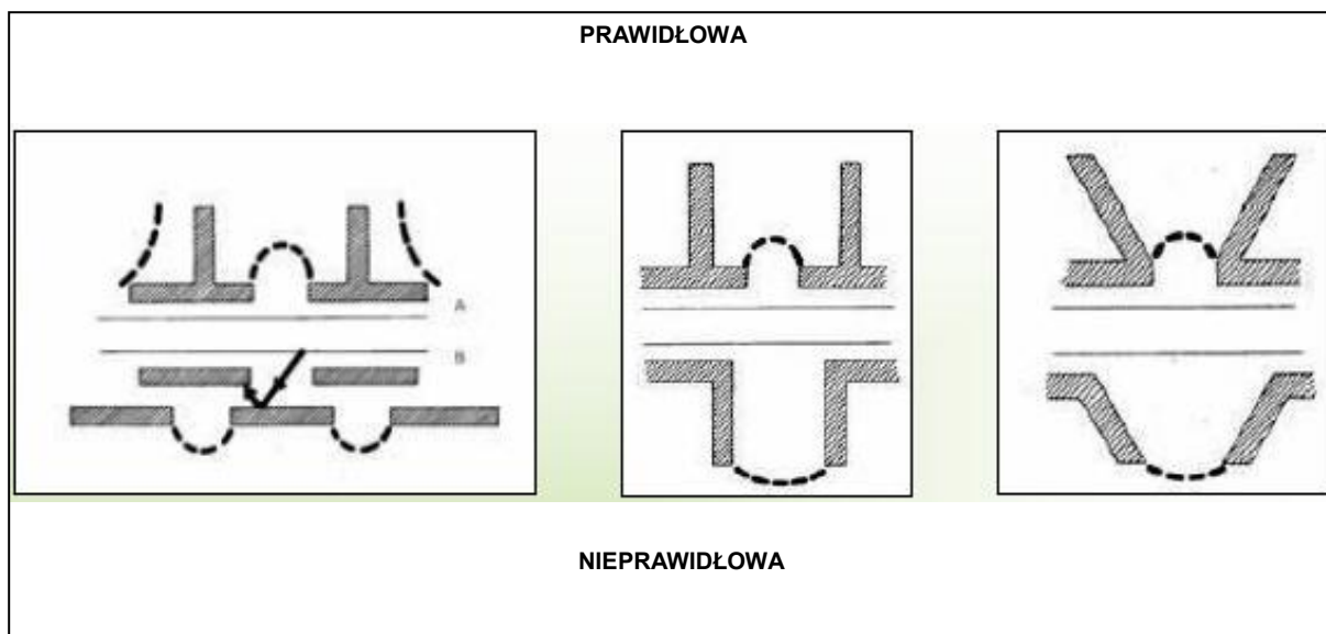
Rys. 9.2. Prawdopodobne i nieprawidłowe orientacje budynków zlokalizowanych w pobliżu drogi, ze względu na wymagania akustyczne
