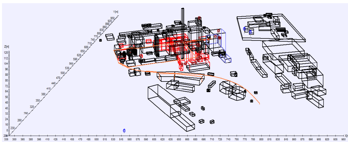
Rysunek 9 Model akustyczny istniejącej części Elektrociepłowni Elbląg oraz obiekty planowanych inwestycji instalacji IOS i SCR
