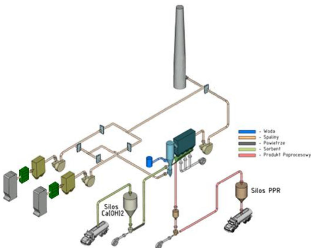
Rysunek 1. Przykładowy schemat instalacji półsuchego odsiarczania spalin – nowy komin
